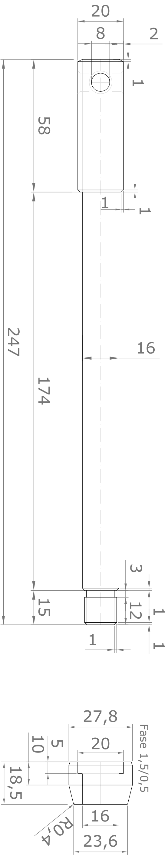
Radachsen und Hülse Victoria KR 26 (N)
