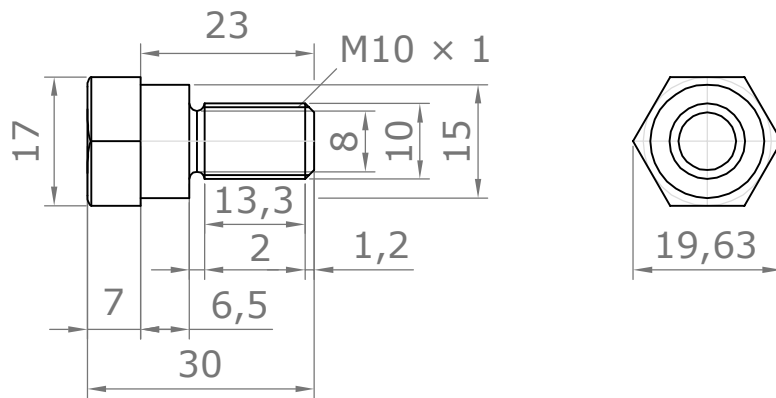
Schraube Hauptständer Victoria KR 26 (N)
